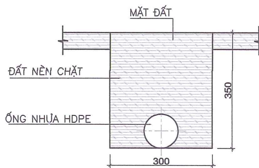
CẮT QUA ỐNG CẤP NƯỚC
