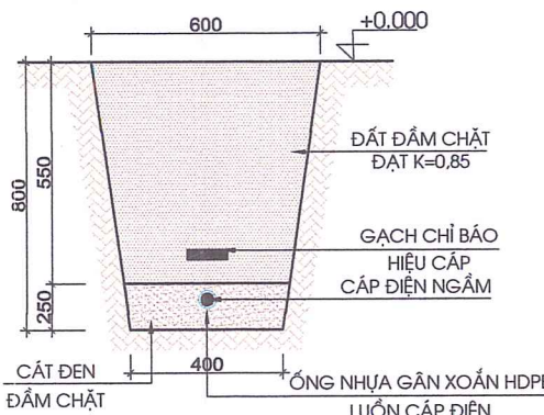
CẮT QUA RÃNH CHÔN CẤP ĐIỆN NGẦM
